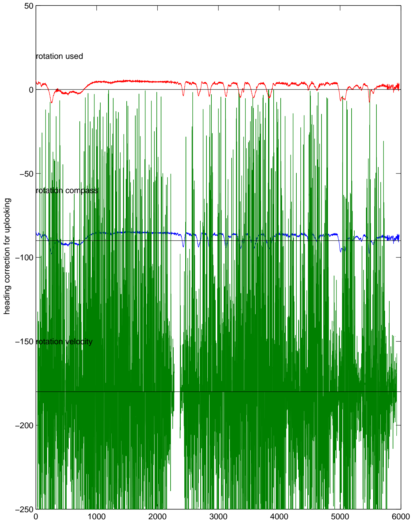
rh10281 (LADCP #036; V5) Figure 5
