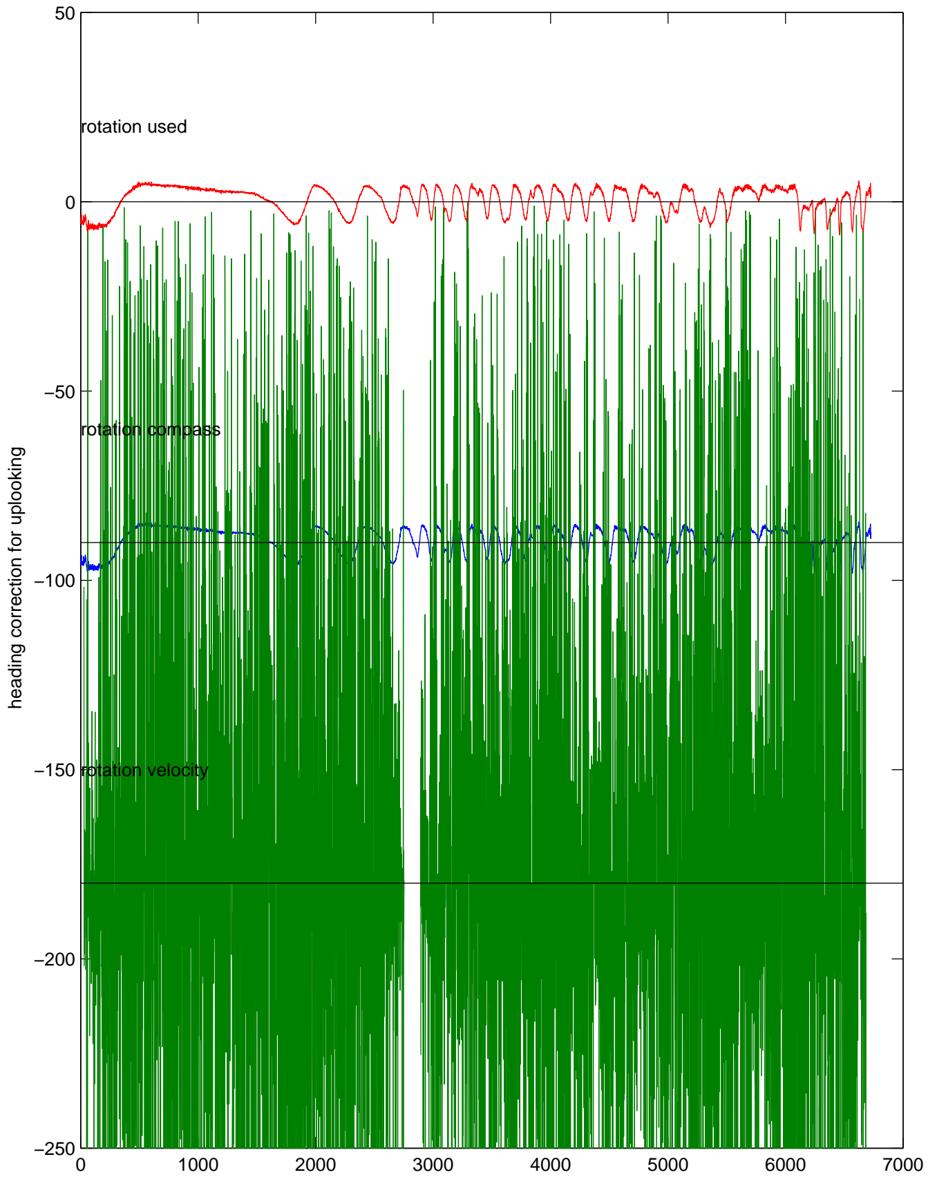
rh10311 (LADCP #039; V5) Figure 5
