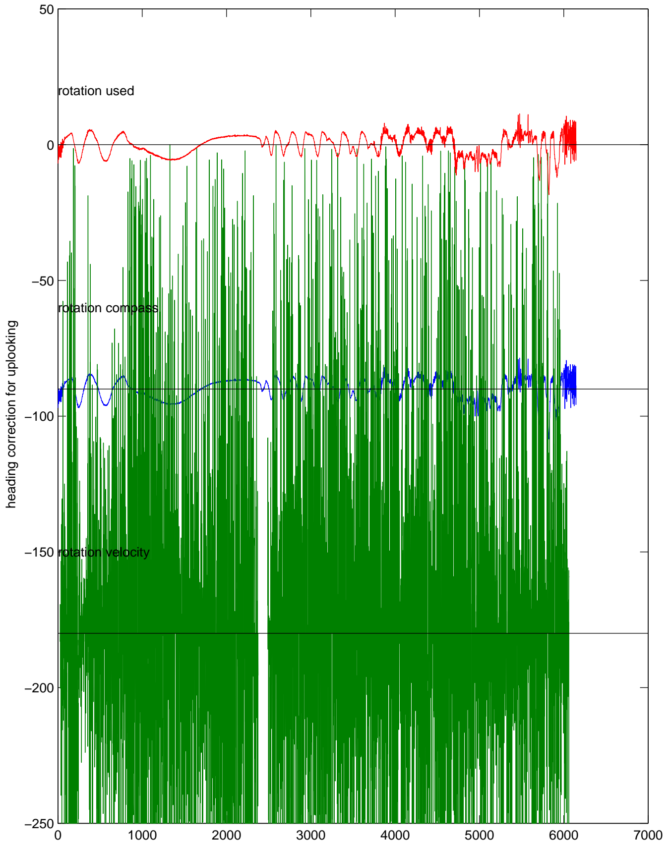
rh10441 (LADCP #052; V5) Figure 5
