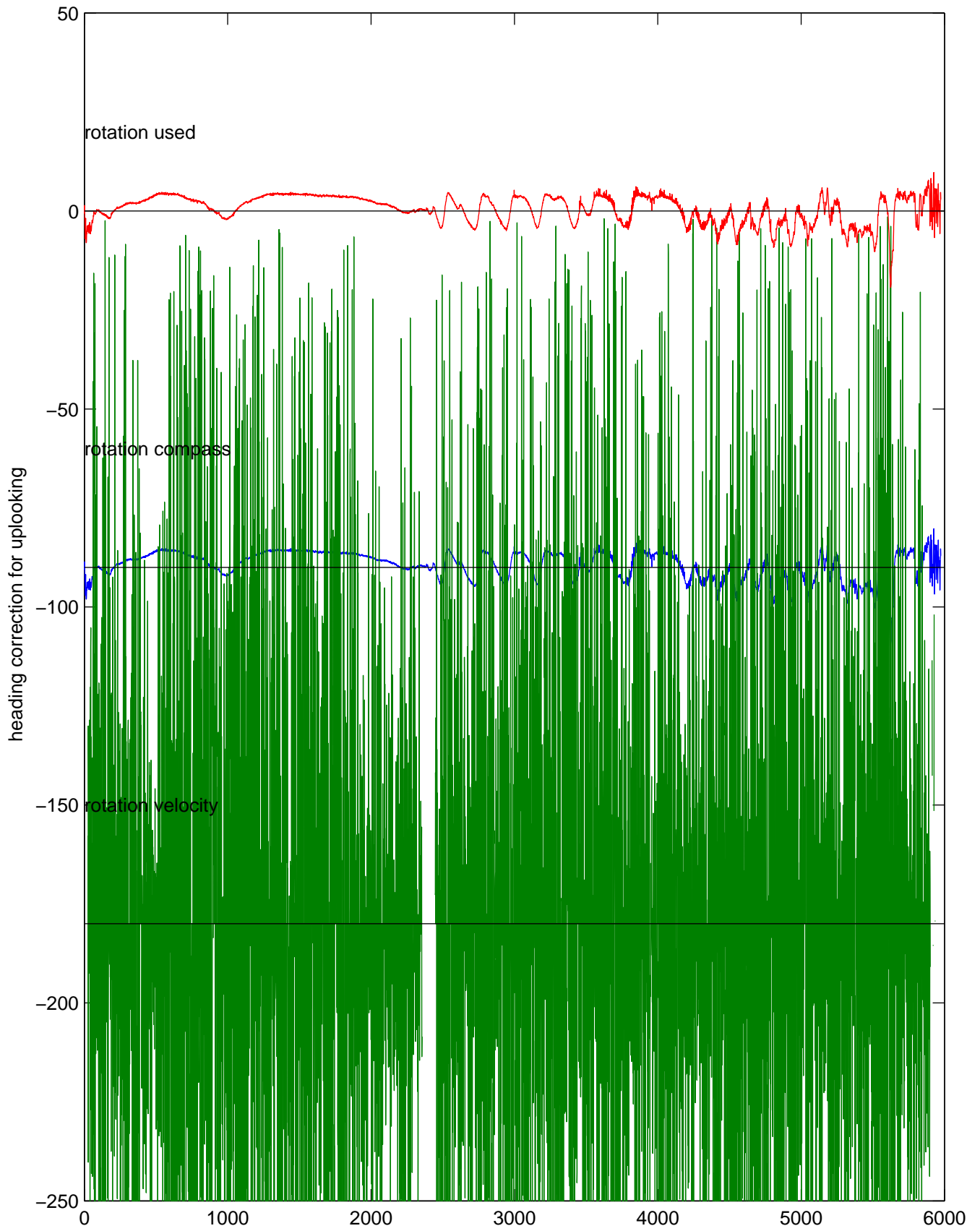
rh10491 (LADCP #057; V5) Figure 5
