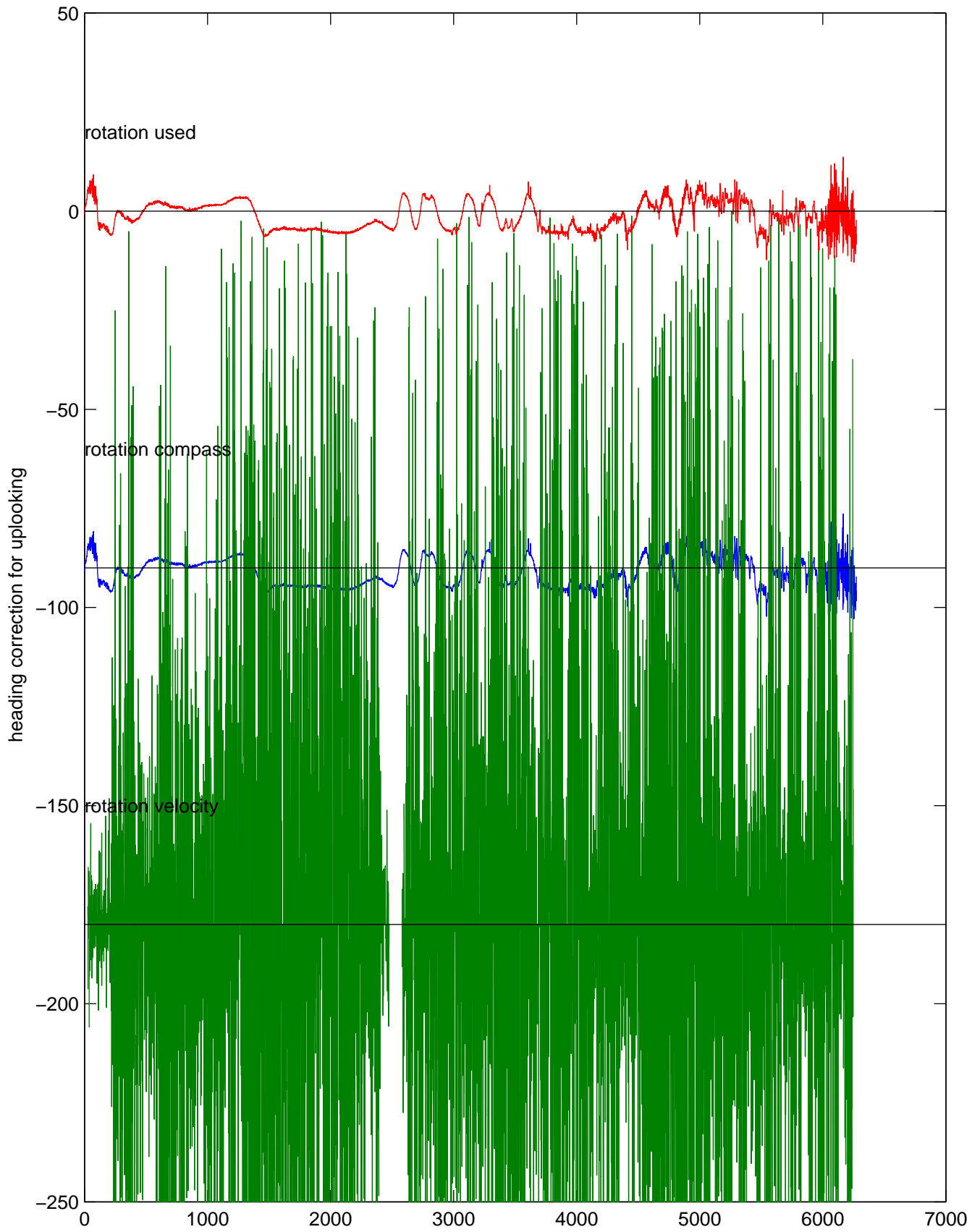
rh10551 (LADCP #063; V5) Figure 5
