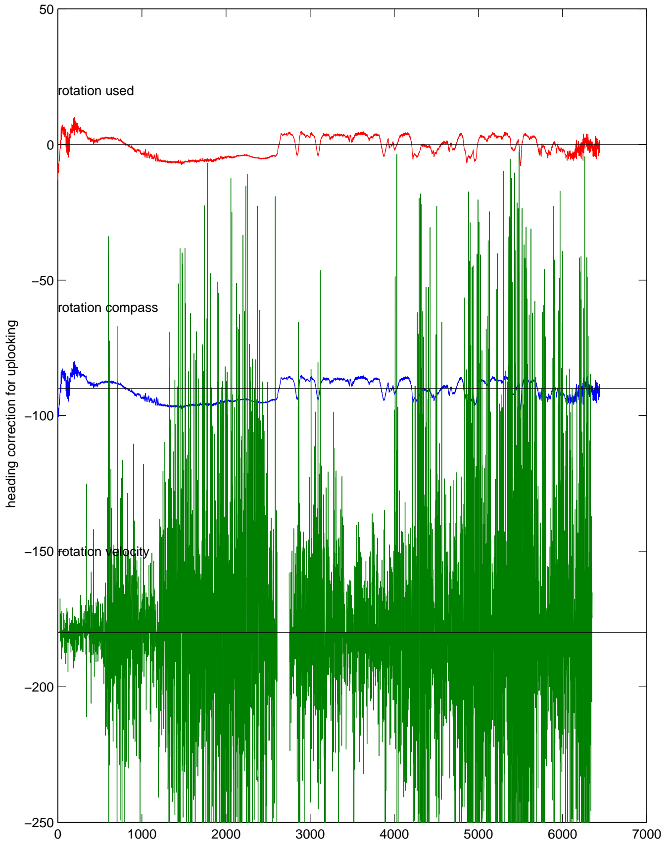
rh10561 (LADCP #064; V5) Figure 5
