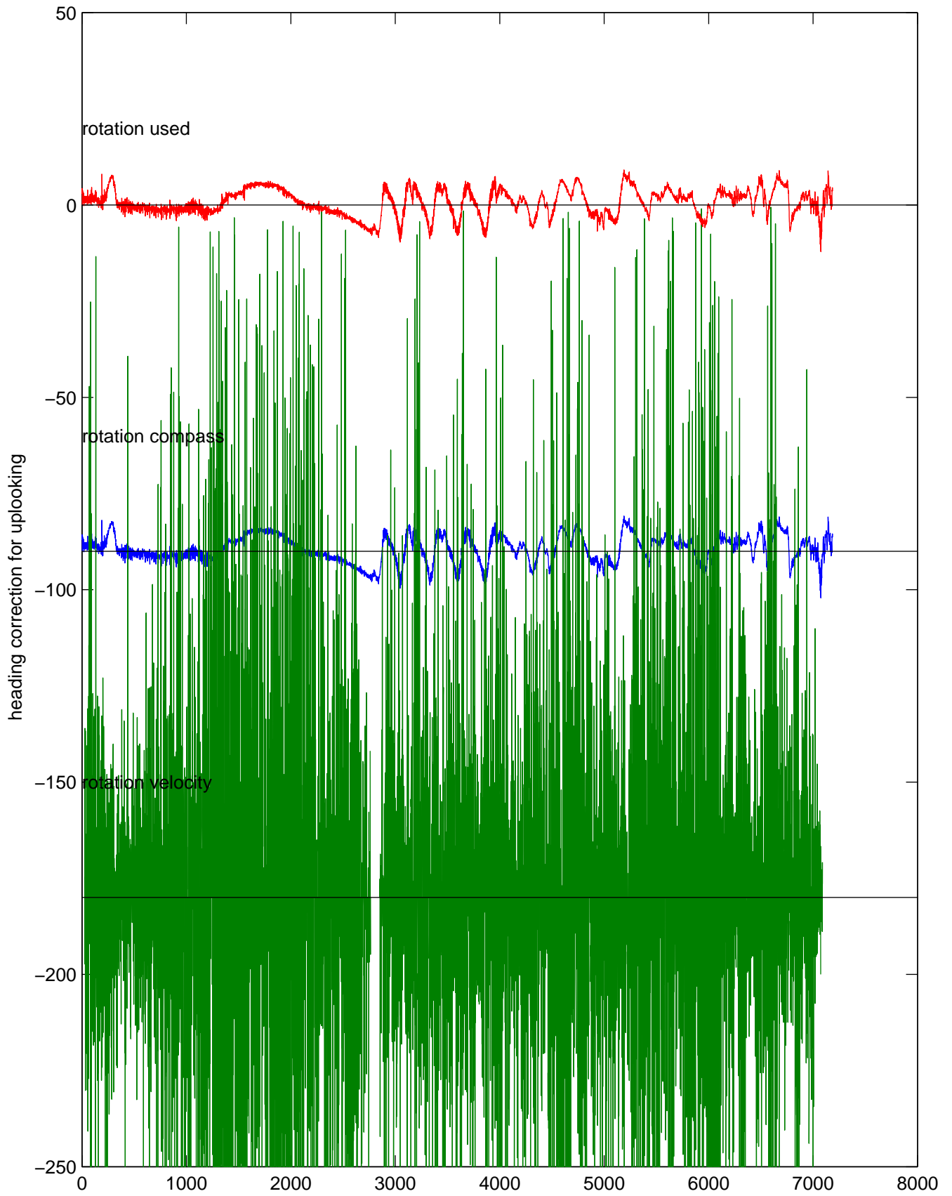
rh11831 (LADCP #196; V5) Figure 5
