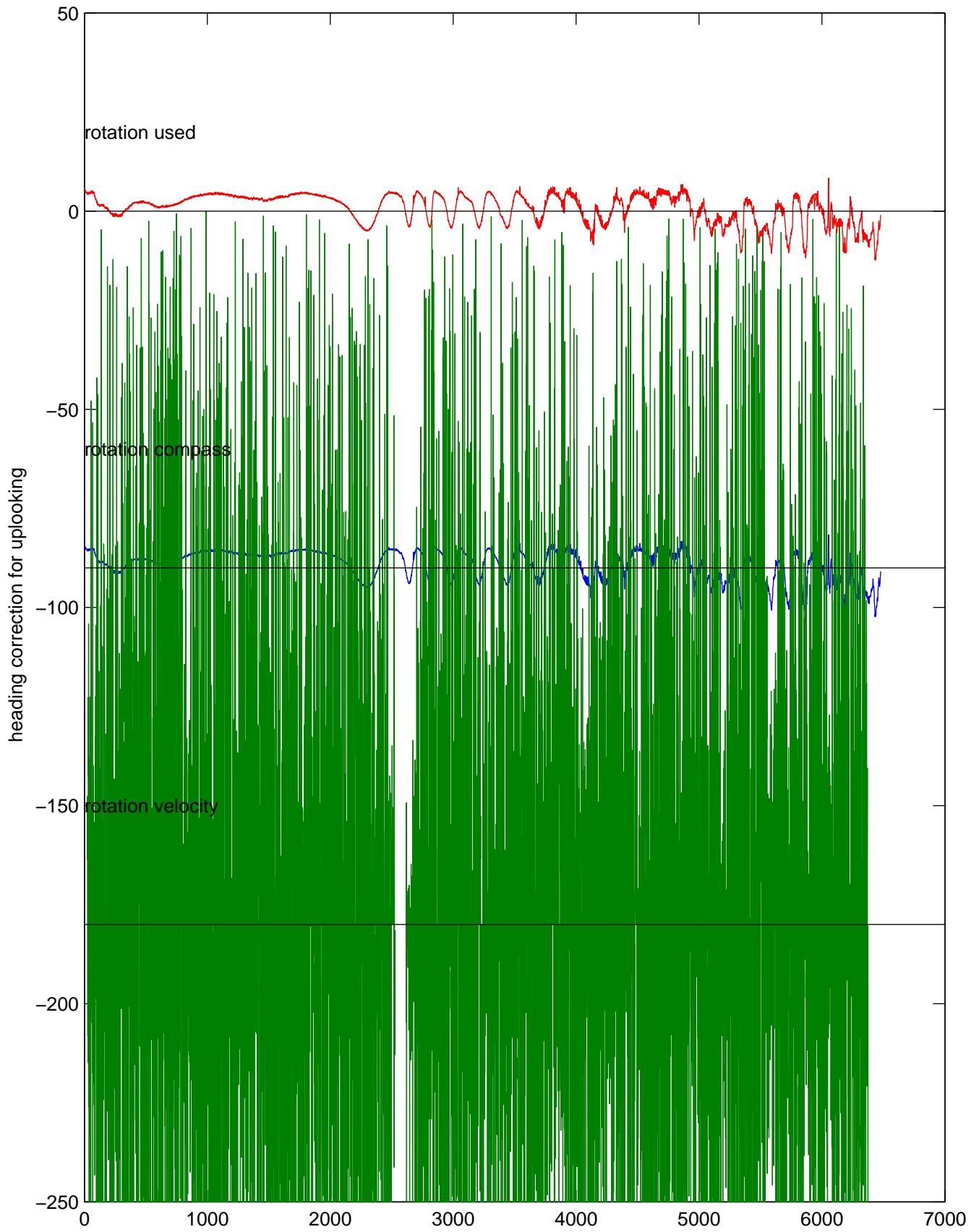
rh10871 (LADCP #095; V5) Figure 5
