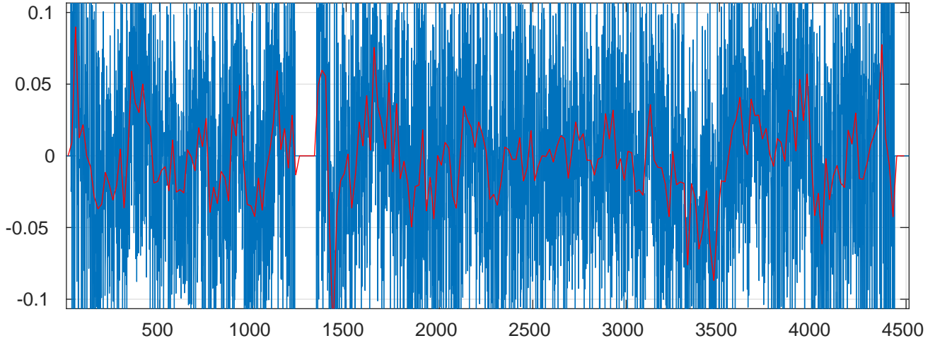
U offset [m/s]
