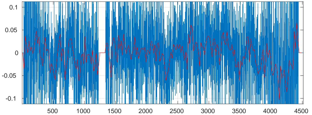
V offset [m/s]
