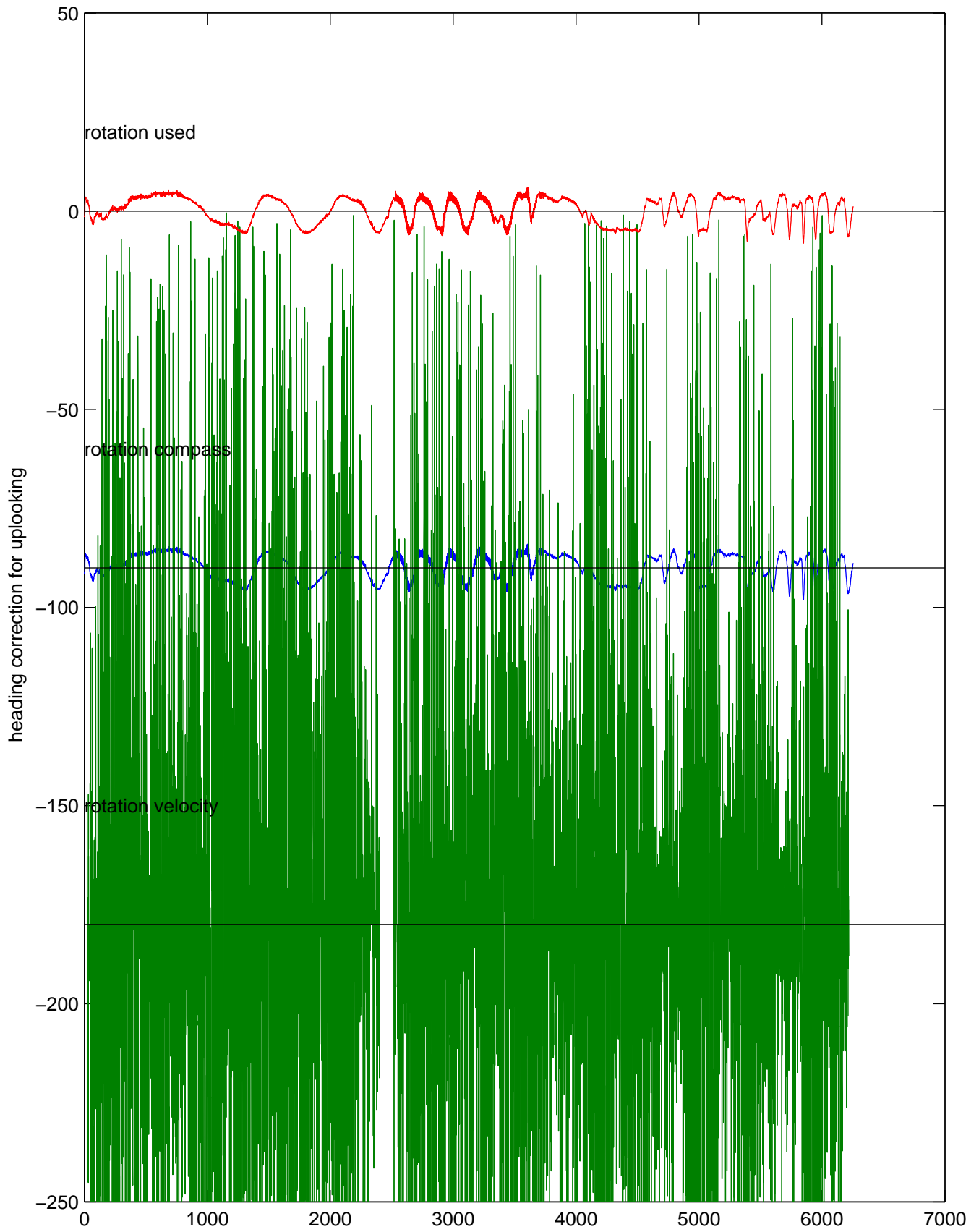
rh10671 (LADCP #075; V5) Figure 5
