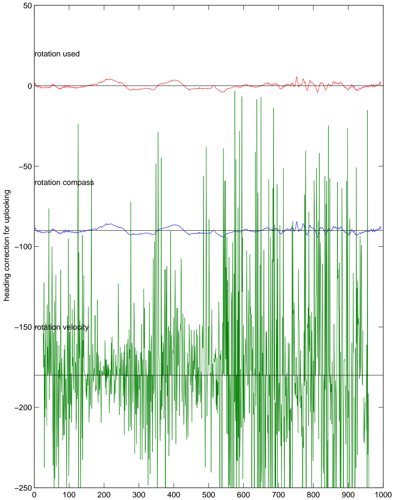
rh10022 (LADCP #009; V5) Figure 5
