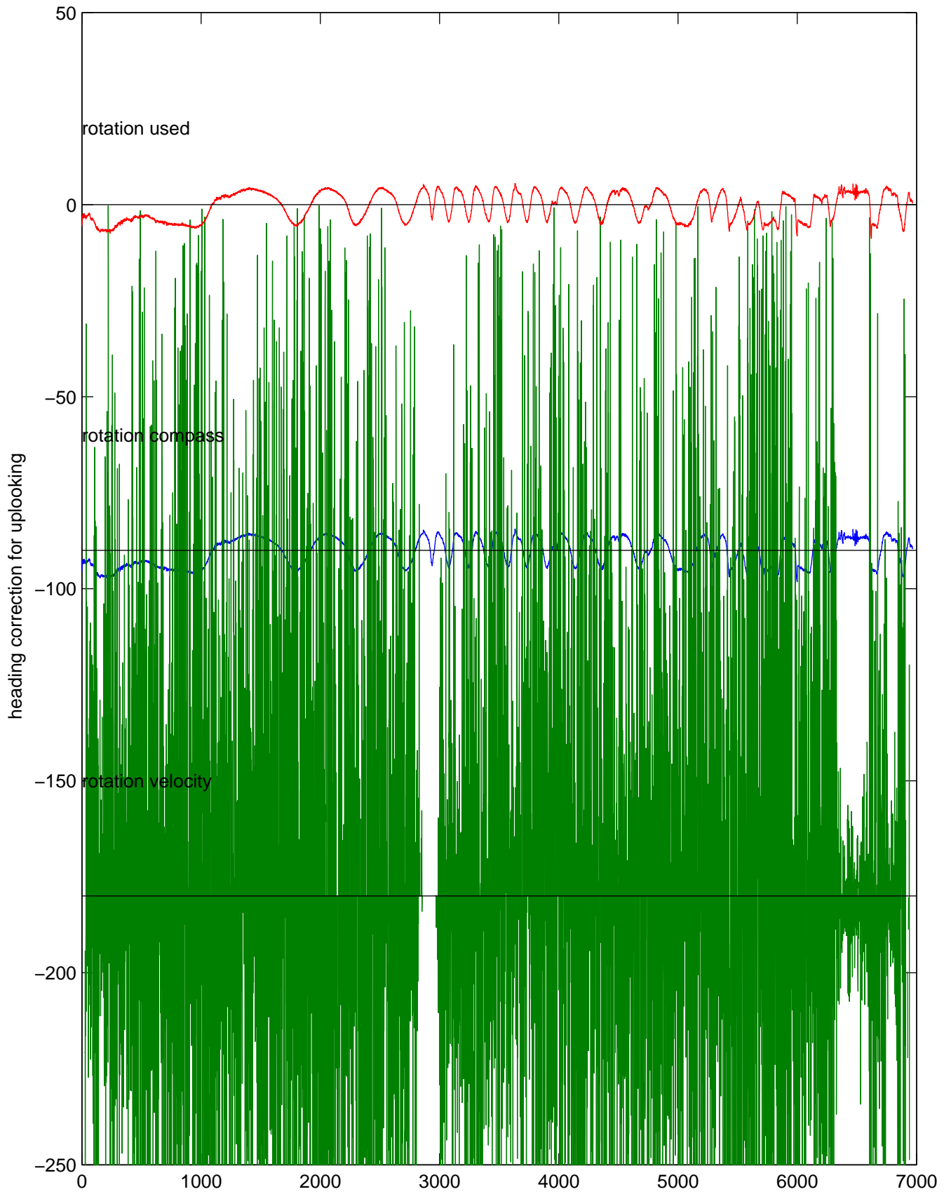
rh10881 (LADCP #096; V5) Figure 5
