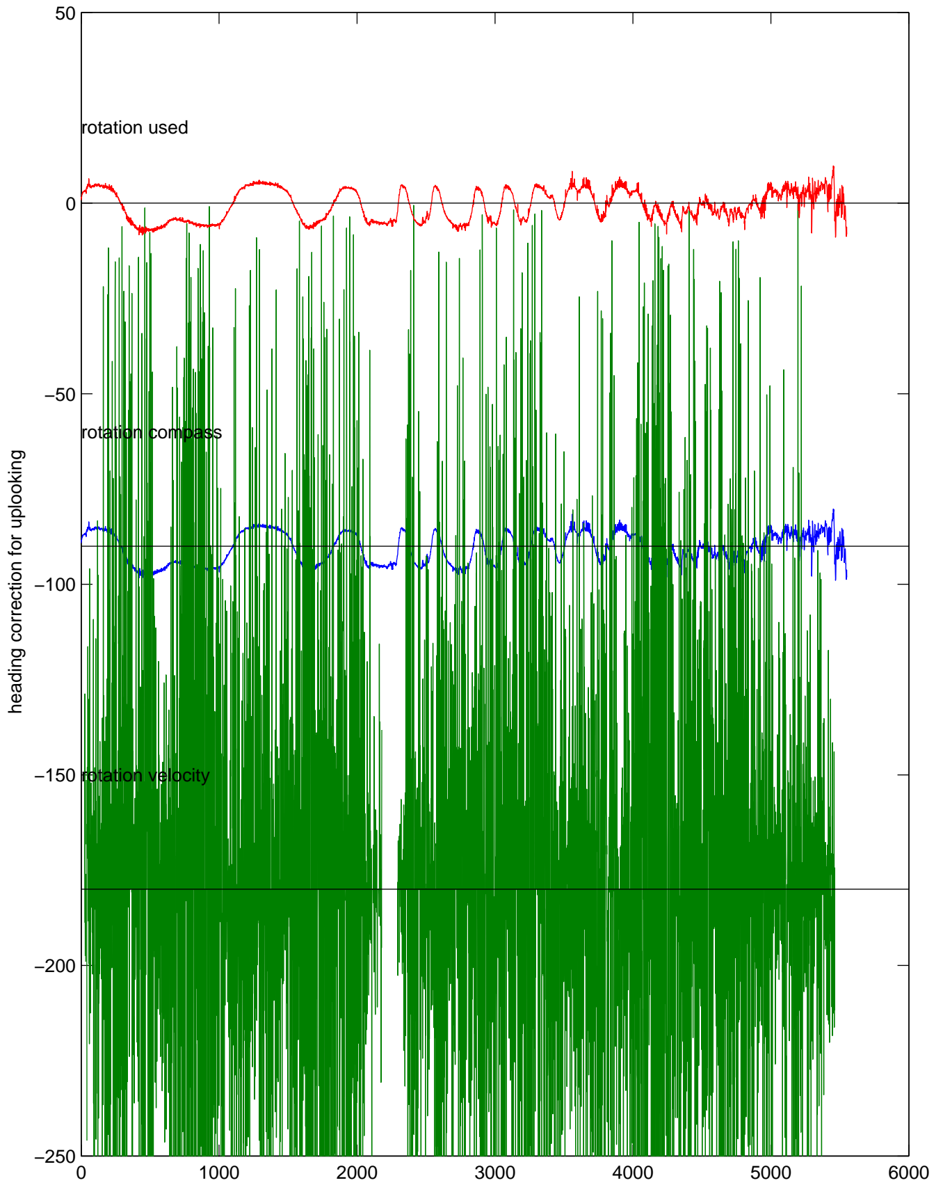
rh10291 (LADCP #037; V5) Figure 5
